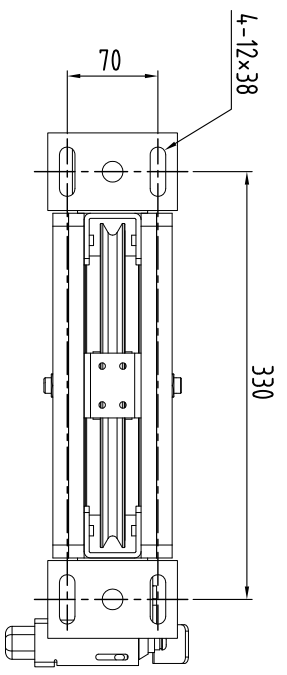
A向视图
