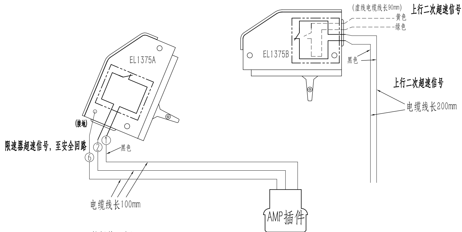
接插件示意图
