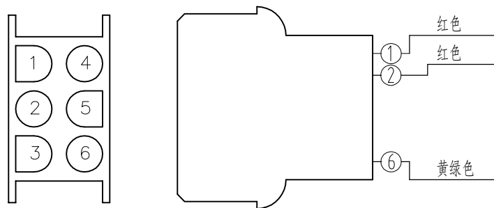
6孔接插线示意图(采用公针)
