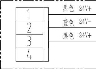
释放电磁铁 (行程开关复位)
