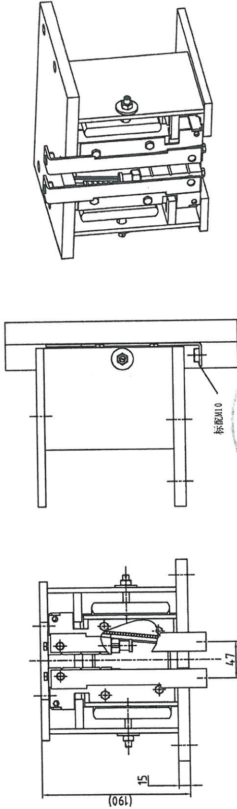
OX-188安全钳 通用 配飞耐导轨
