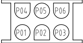
6孔接插线示意图(采用母针)
