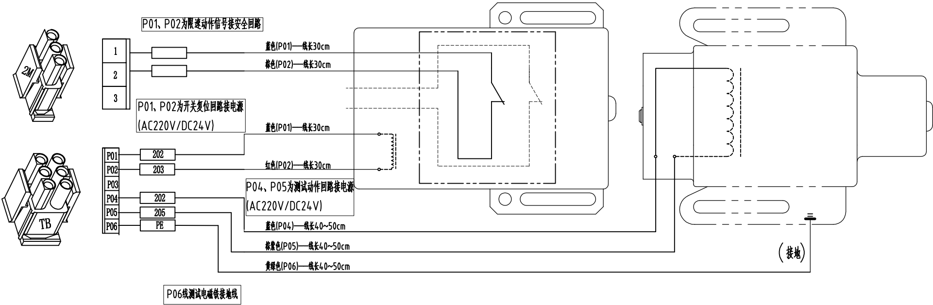
3孔接插线示意图(采用母针)
