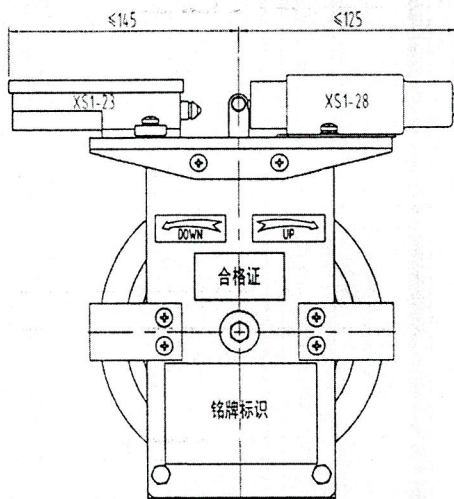
A向视图
