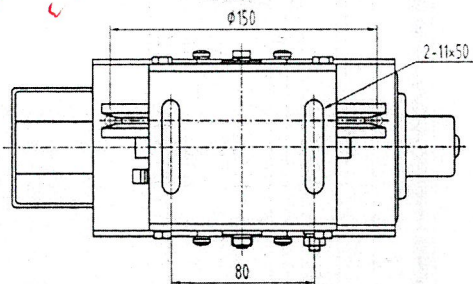
A向视图
