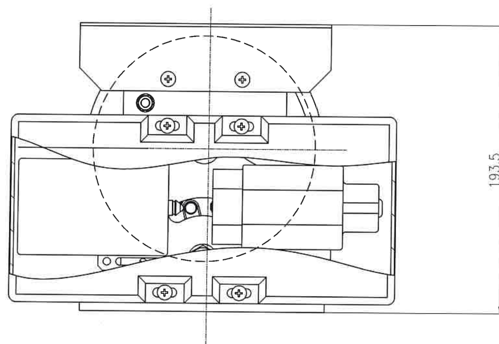
限速器安装尺寸示意图
