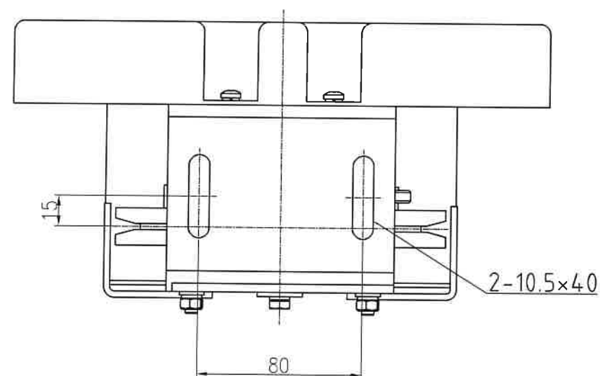
限速器安装尺寸示意图
