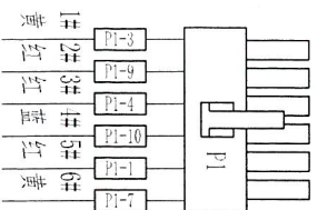
接插件接线示意图
