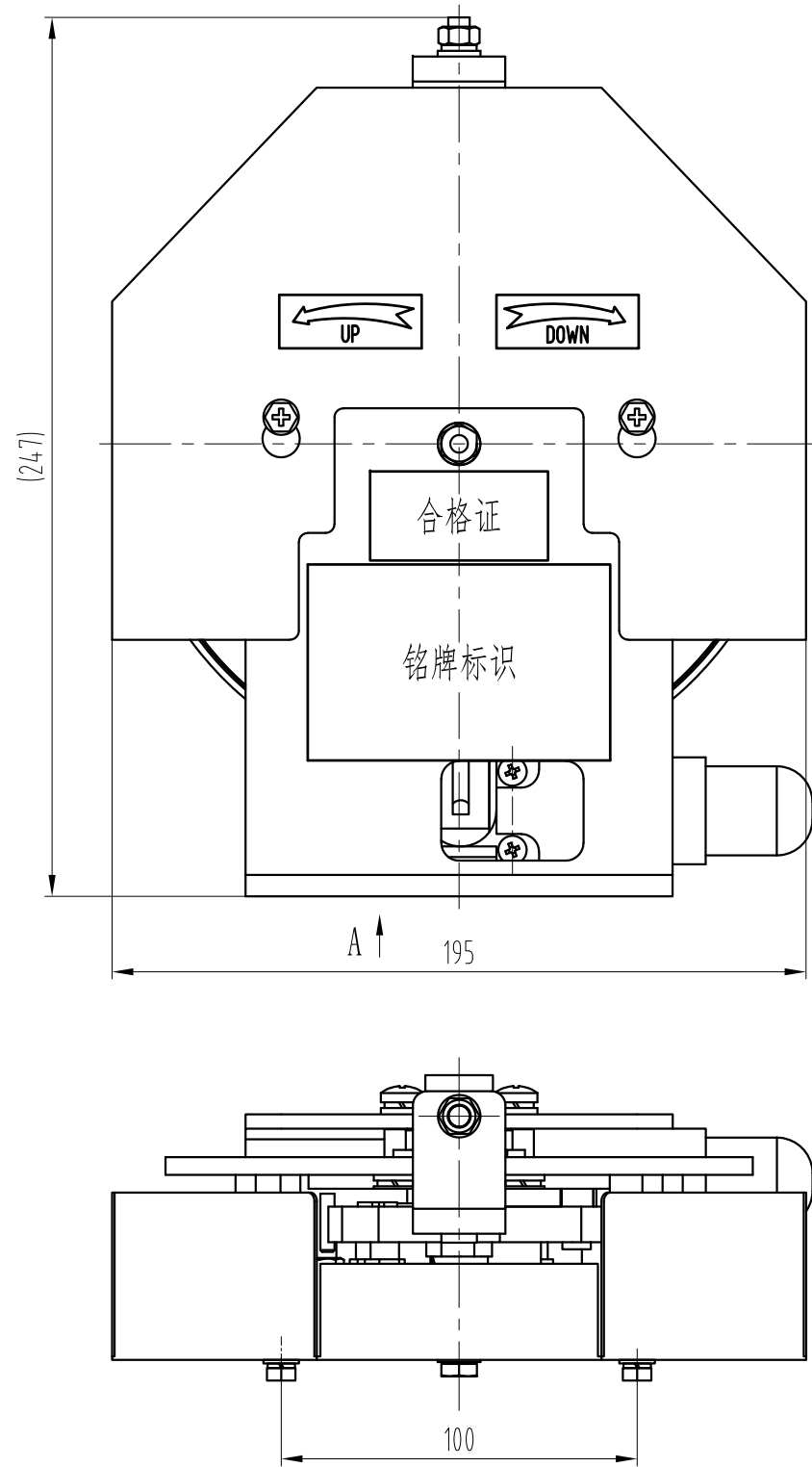
左置式(常规)
