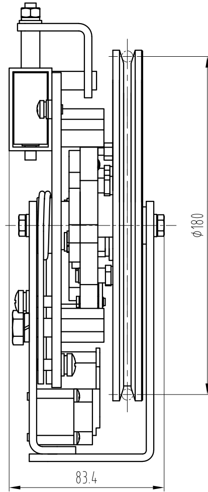
视图A 80
