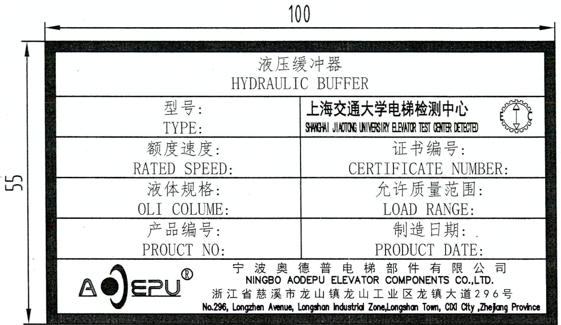
图示为缓冲器奥德普铭牌(G01时使用, 材质不干胶) 型式试验编号: TSX F33002220220069
