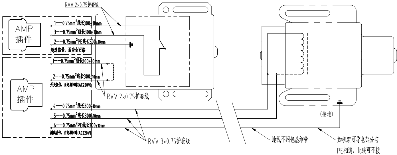
无机房限速器开关接线示意图
