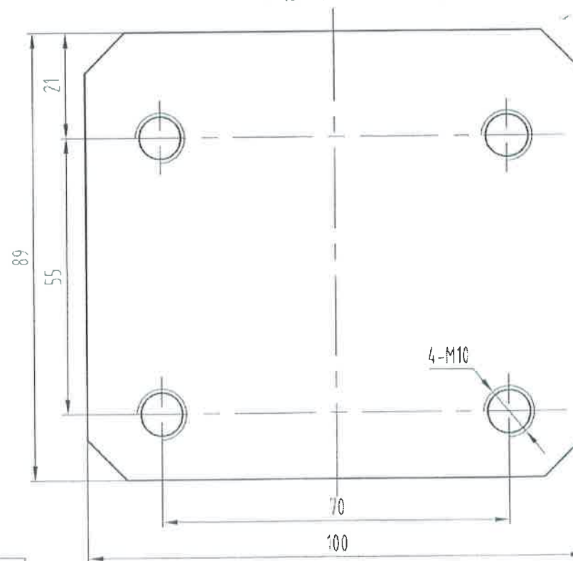
B (安装孔示意图)
