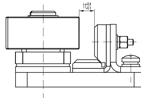
B (安装孔示意图)
