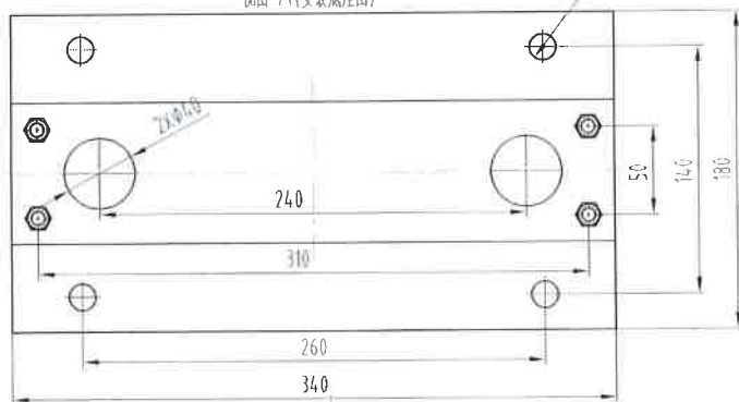
视图 A (安装底座图)
