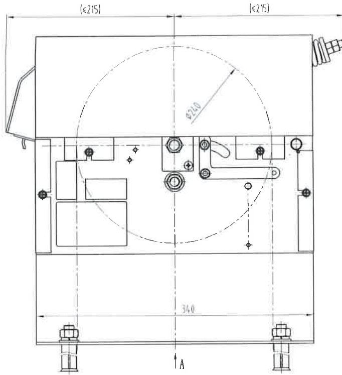
A(安装孔)
