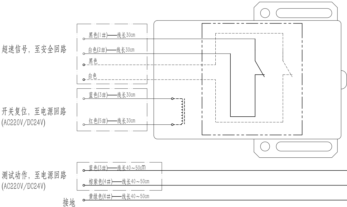
XS1-23接线示意
