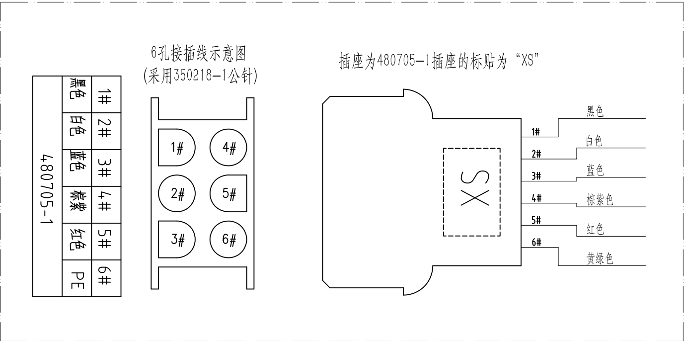
线号示意（接插件时）
