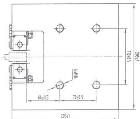
导轨安装面 A 180°
