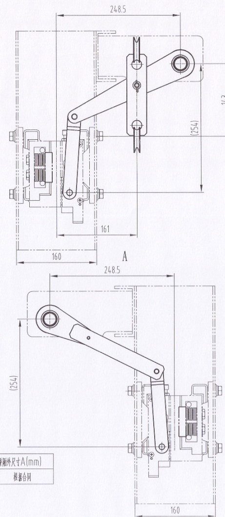
UKT开关 1件 十字槽小盘头螺钉 GB/T 823 M4×40 2件 六角螺母 GB/T 6170 M4 2件 弹性圆柱销 GB/T 879.4/6×12 2件
