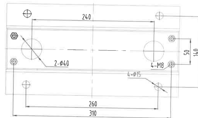
视图 A
