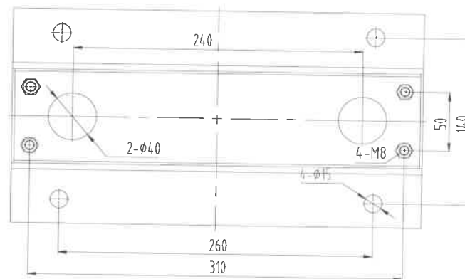
视图 A
