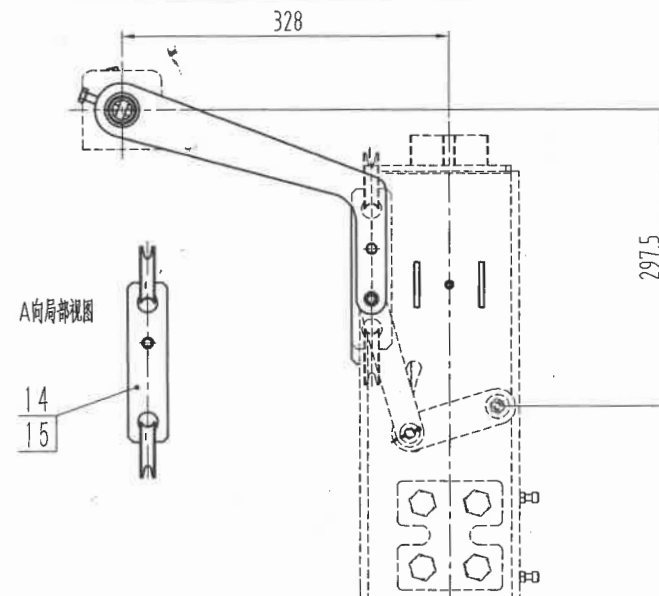
89200165 OX-210CT(XA02)安全联动装置 DBG=640mm 镀白锌 中英文包装 左提拉 杭州西奥(镀彩锌)V3
