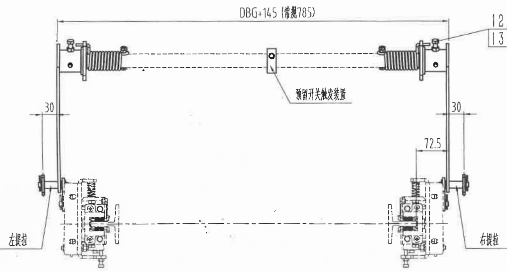
89200164 OX-210CT(XA02)安全联动装置 DBG=640mm 镀白锌 中英文包装 右提拉 杭州西奥(镀彩锌)
