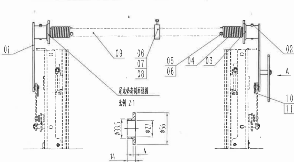
89200164 OX-210CT(XA02)安全联动装置 DBG=640mm 镀白锌 中英文包装 右提拉 杭州西奥(镀彩锌)
