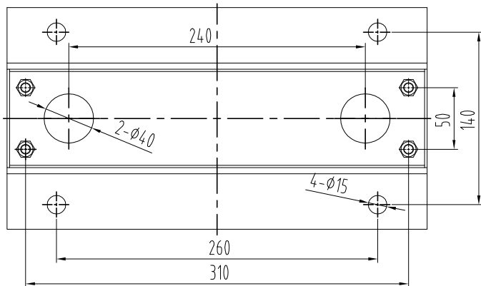
A向视图
