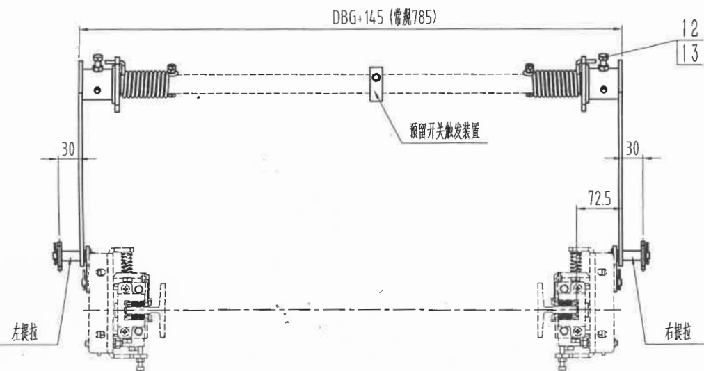
89100108 OX-210CT(XA02)安全联动装置 DBG=640mm 镀白锌 中英文包装 右提拉 杭州西奥
