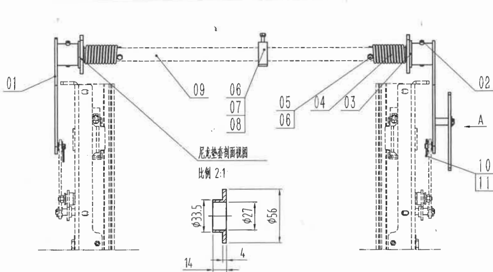
89100108 OX-210CT(XA02)安全联动装置 DBG=640mm 镀白锌 中英文包装 右提拉 杭州西奥
