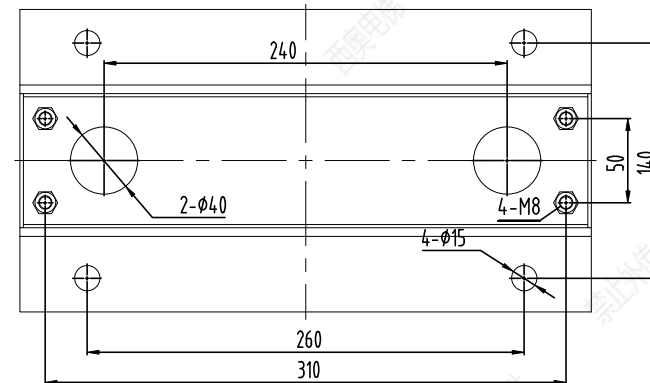
视图 A
