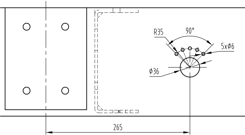
开孔示意图
