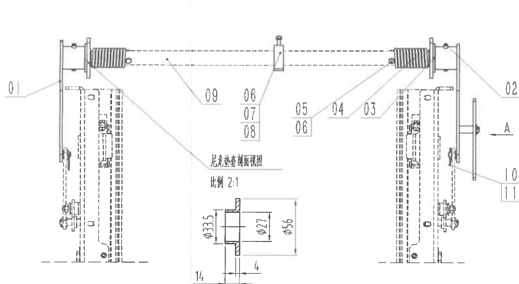
89100032 OX-210CT(XA02)安全联动装置 DBG=785mm 中英文包装 左提拉 杭州西奥
