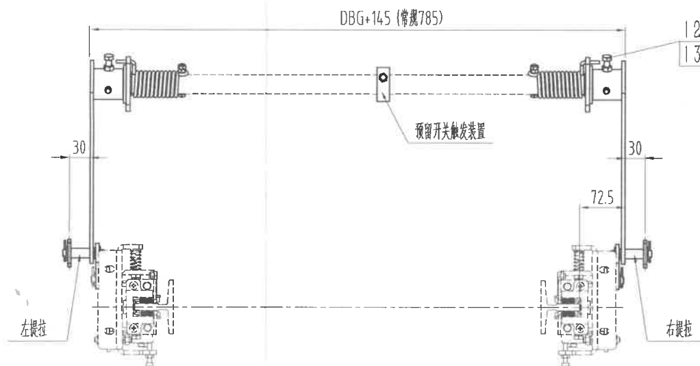
89100032 OX-210CT(XA02)安全联动装置 DBG=785mm 中英文包装 左提拉 杭州西奥
