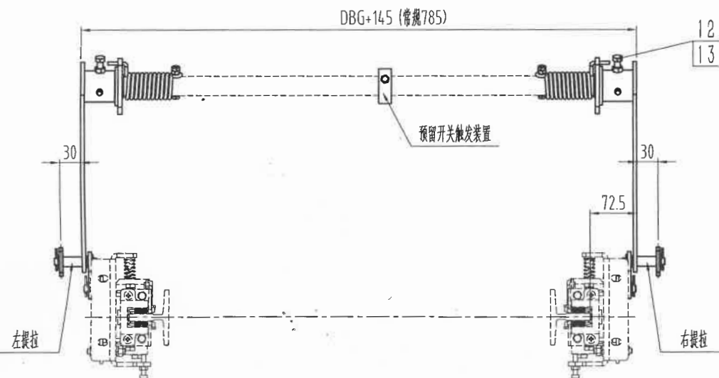
89100032 OX-210CT(XA02)安全联动装置 DBG=640mm 镀白锌 中英文包装 左提拉 杭州西奥 V3
