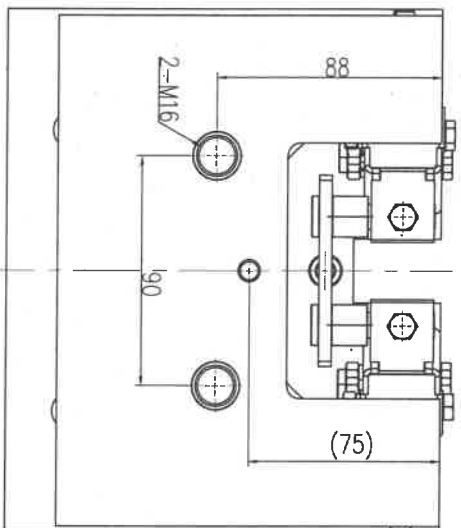
视图 A
