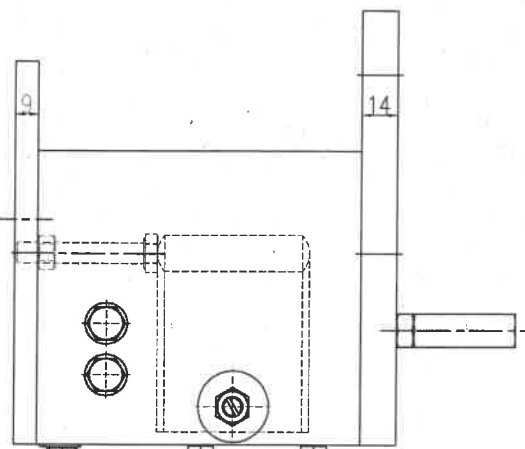
视图 A
