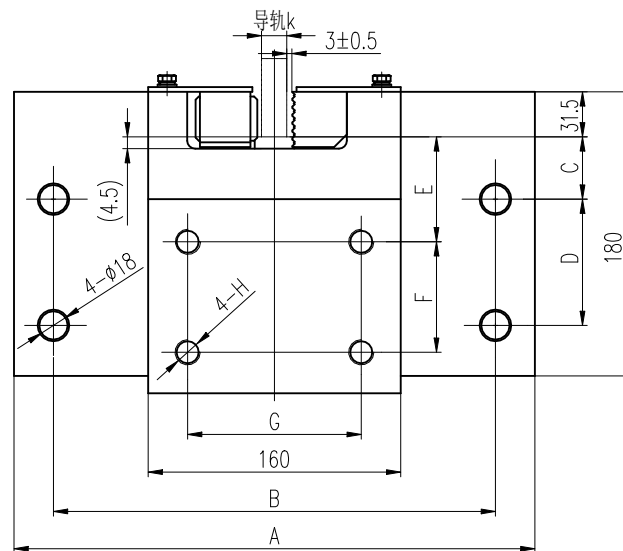
A向视图
