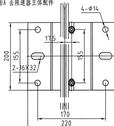
视图A 去限速器主体配件
