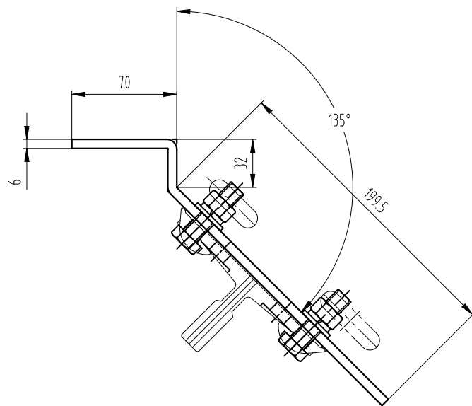
A向视图
