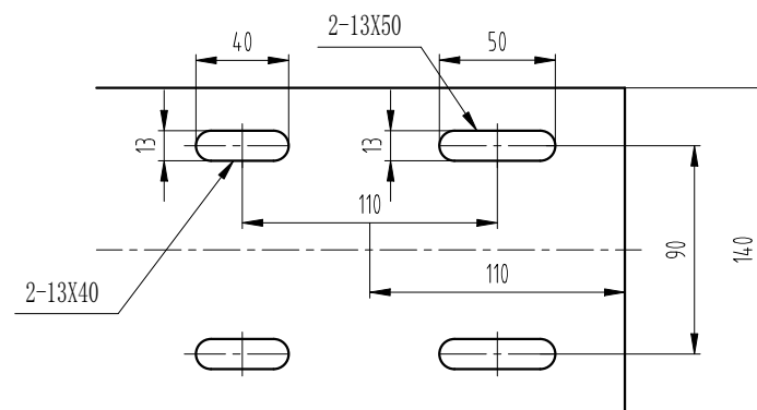
A向视图
