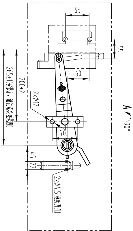
开孔尺寸
