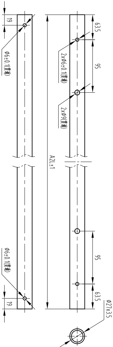
连接圆管开孔图
