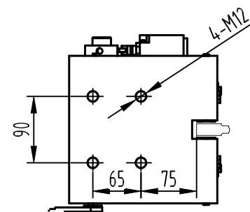
A视图, 导靴安装孔位
