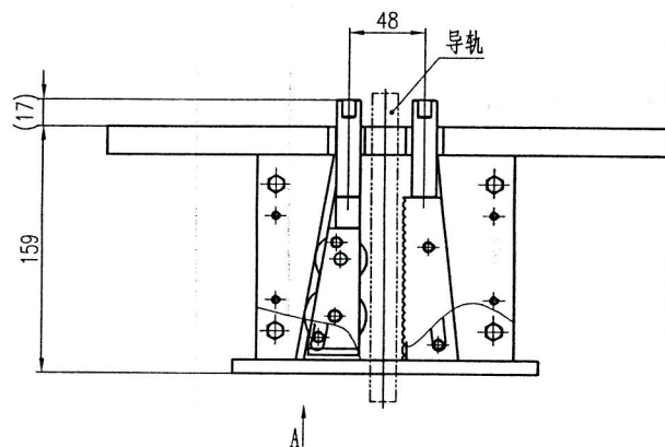
A向视图
