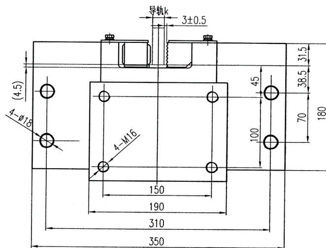
A向视图
