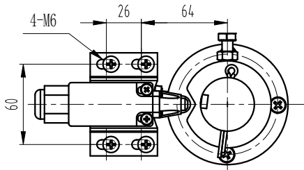
下梁开关安装座开孔尺寸
