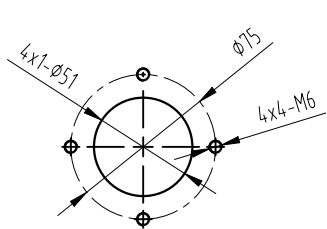
下梁转轴开孔尺寸
