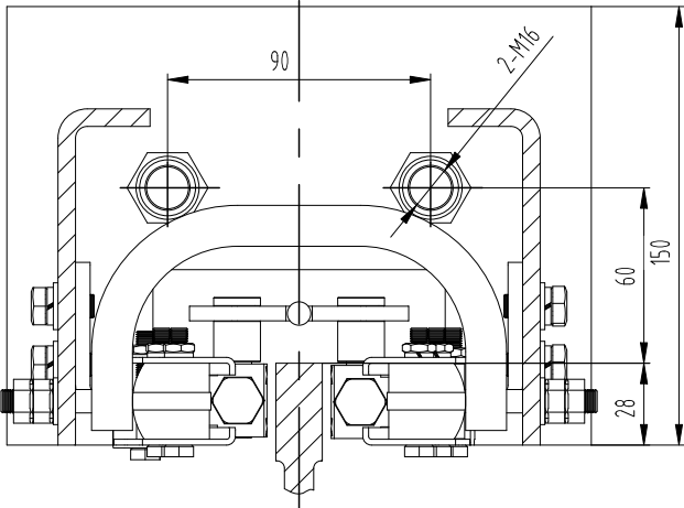
A向视图
