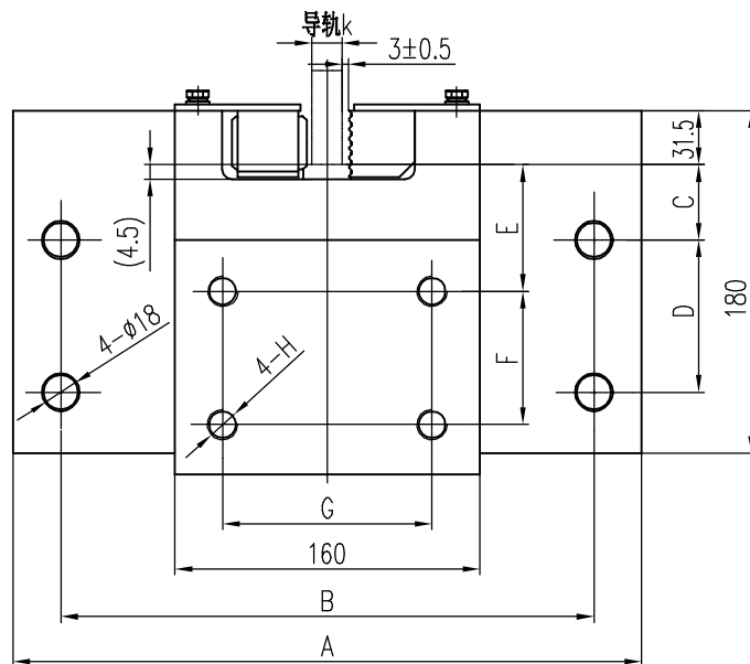
A向视图
