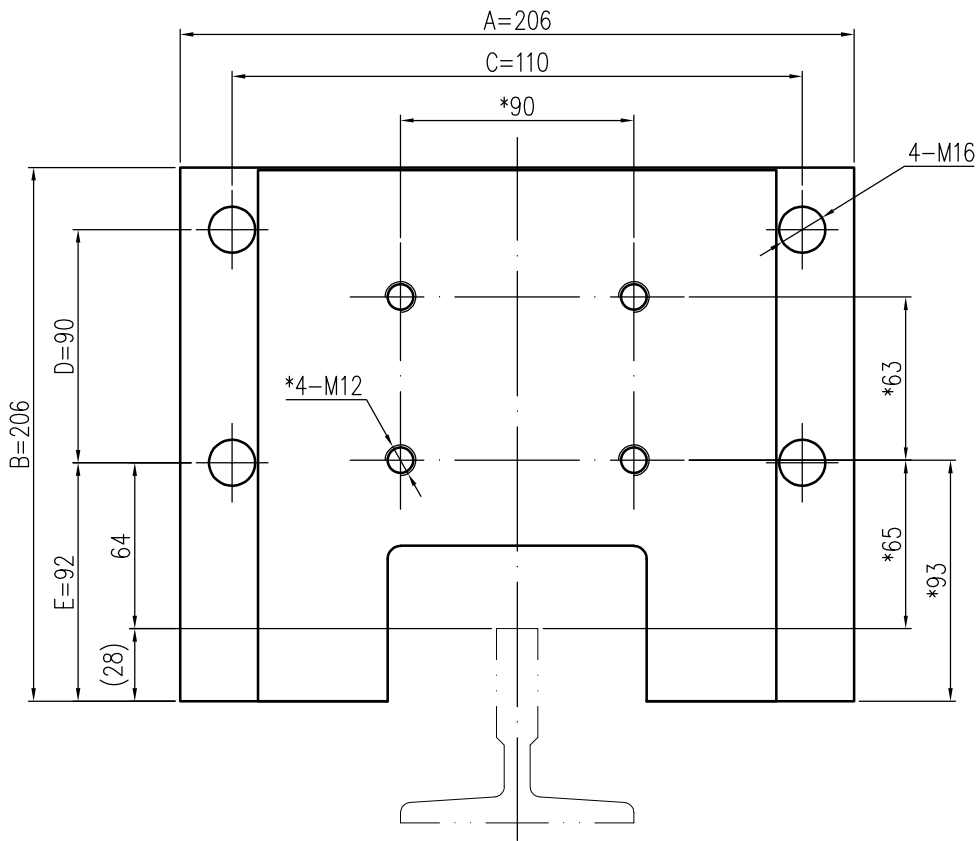
连接孔位示意图
