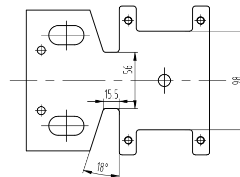
展开示意图
