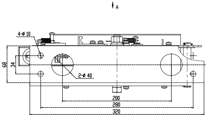
视图 A
