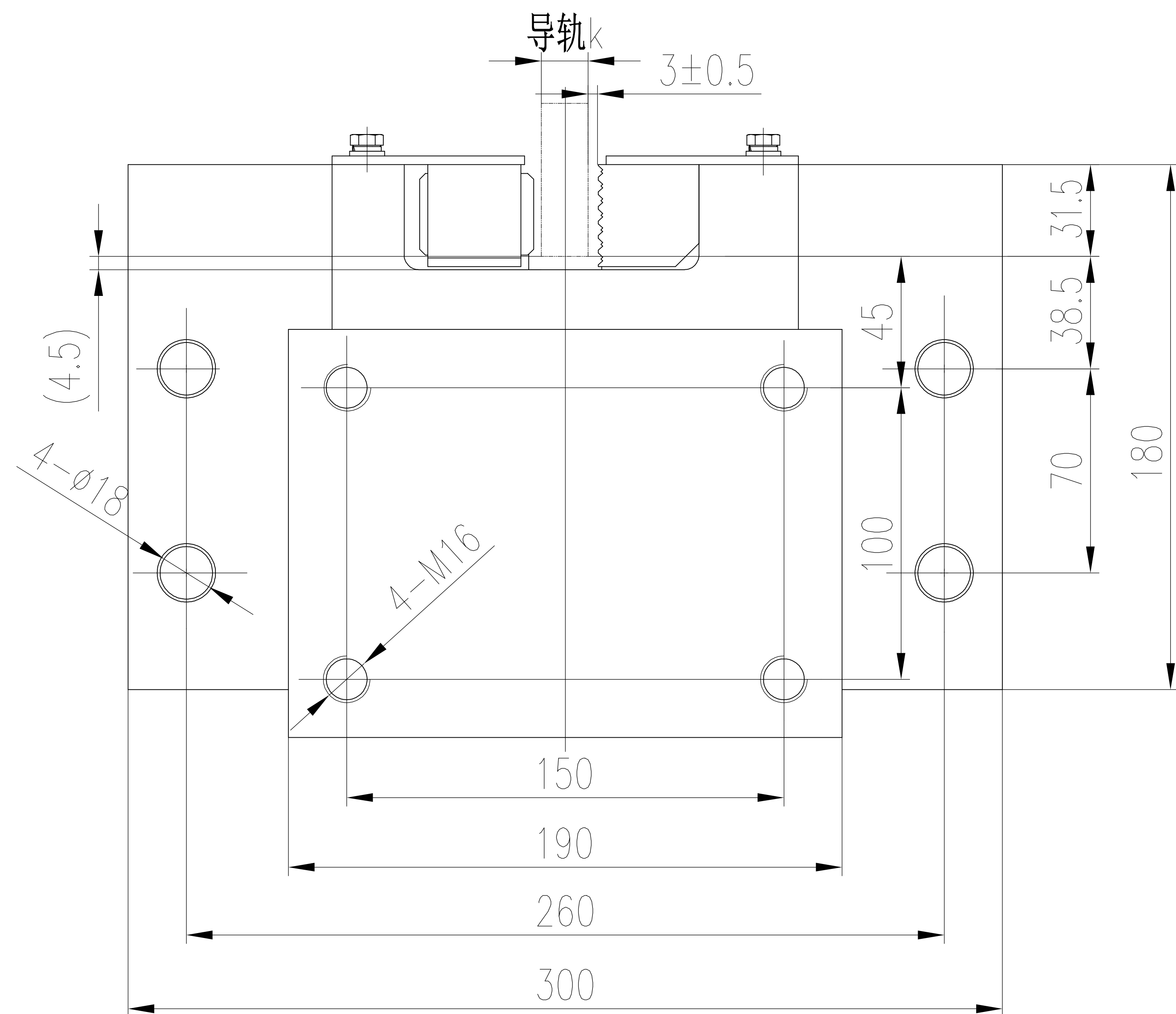
A向视图
