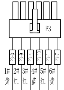
接插件接线示意图
