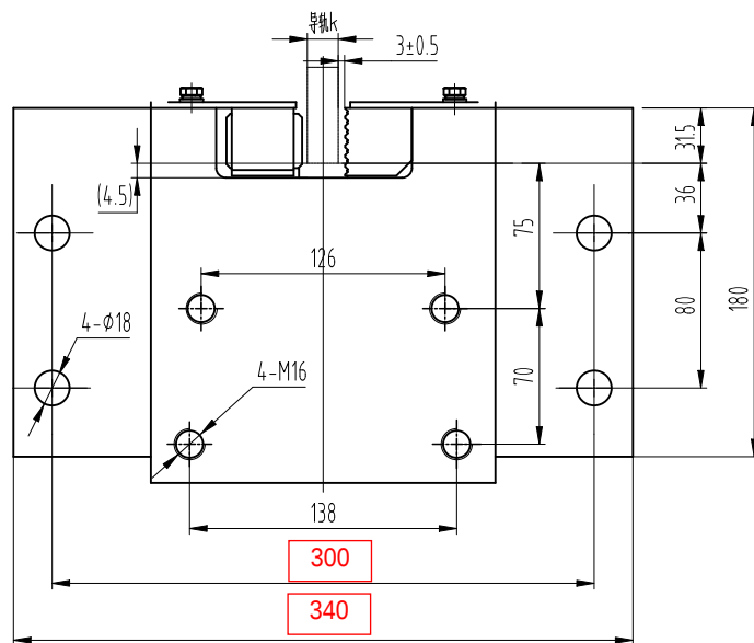
A向视图
