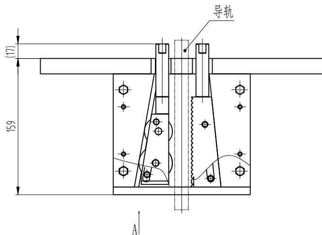
A向视图
