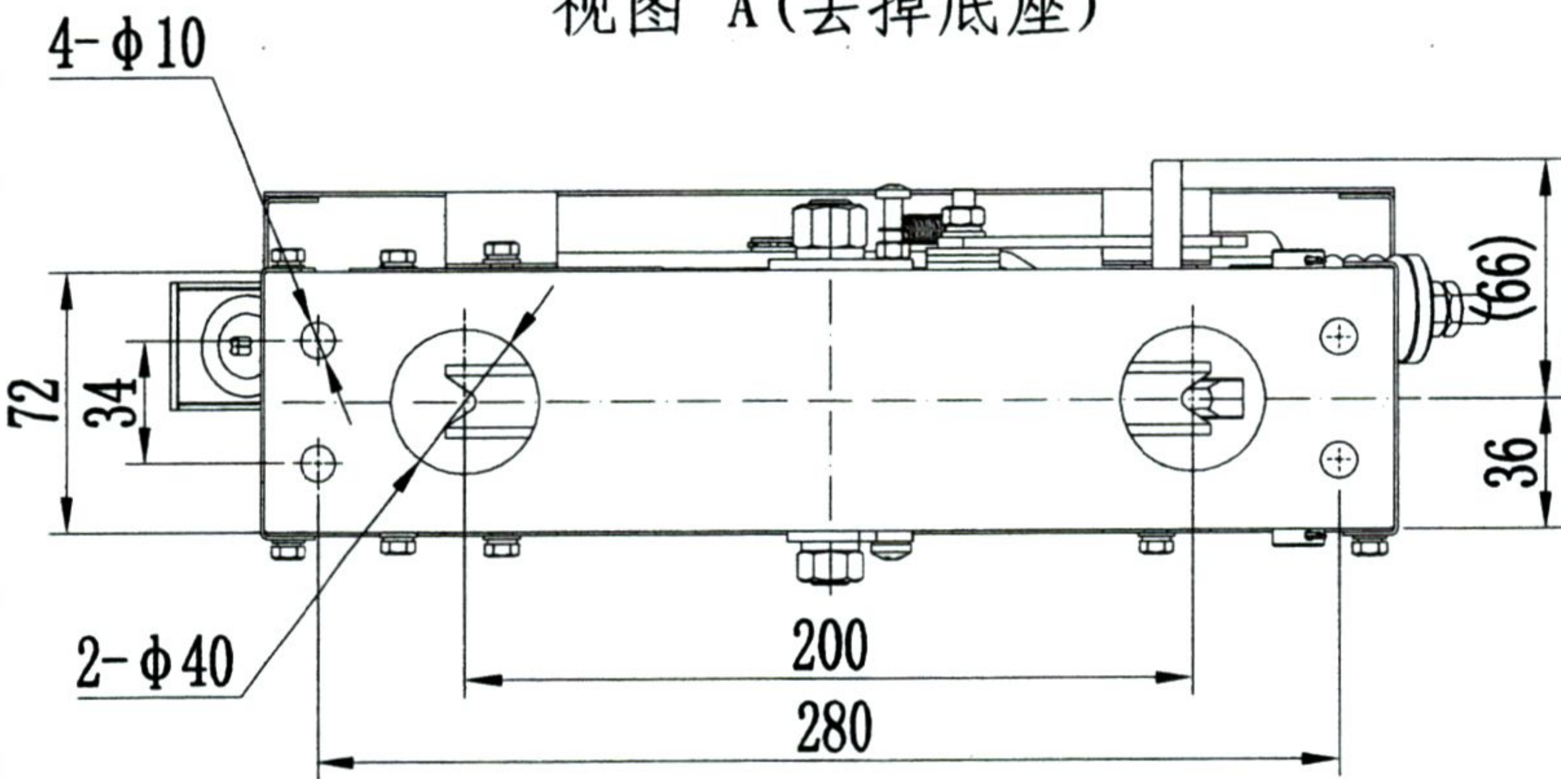
视图 A (去掉底座)
