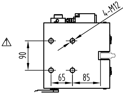
A视图，导轨安装孔位
