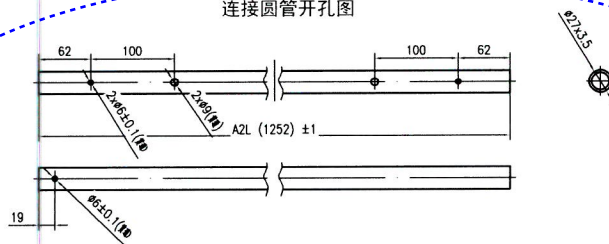
连接圆管开孔图
