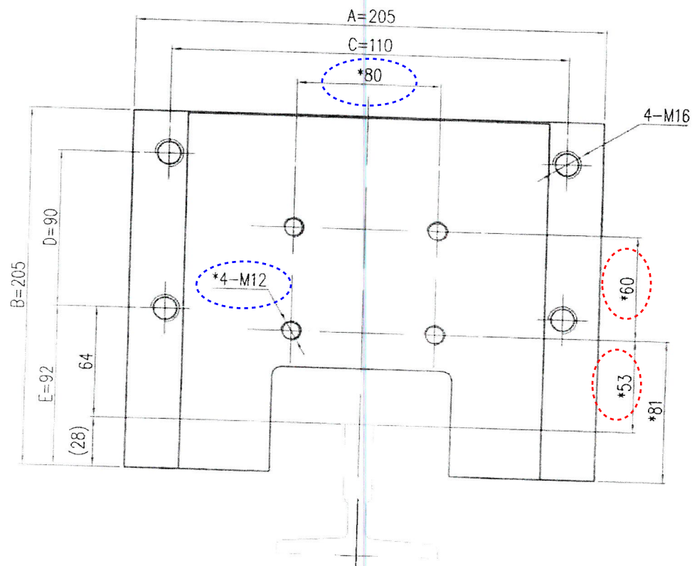
连接孔位示意图
