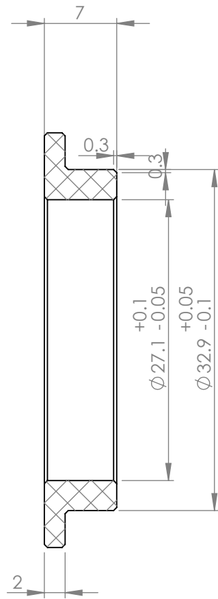
SECCIÓN B-B
