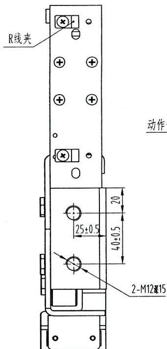
接插件接线示意图
