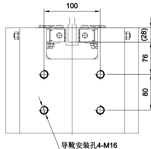
B视图
